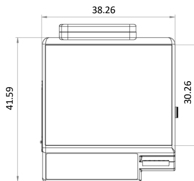
Vista lateral
